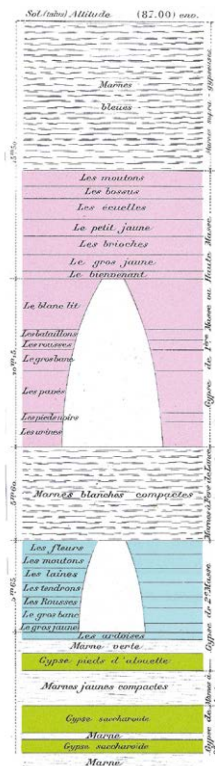
Coupe de terrain à Villemomble
