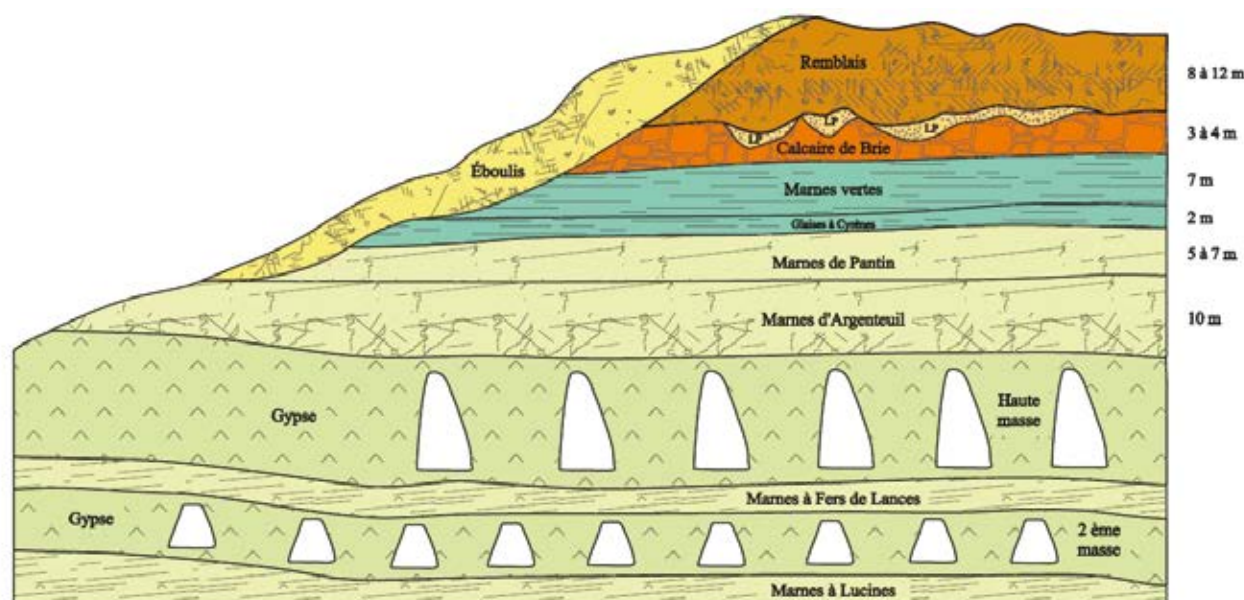
Coupe géologique schématisée de la commune
