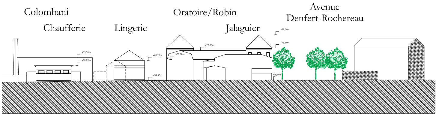
COUPE CC'
