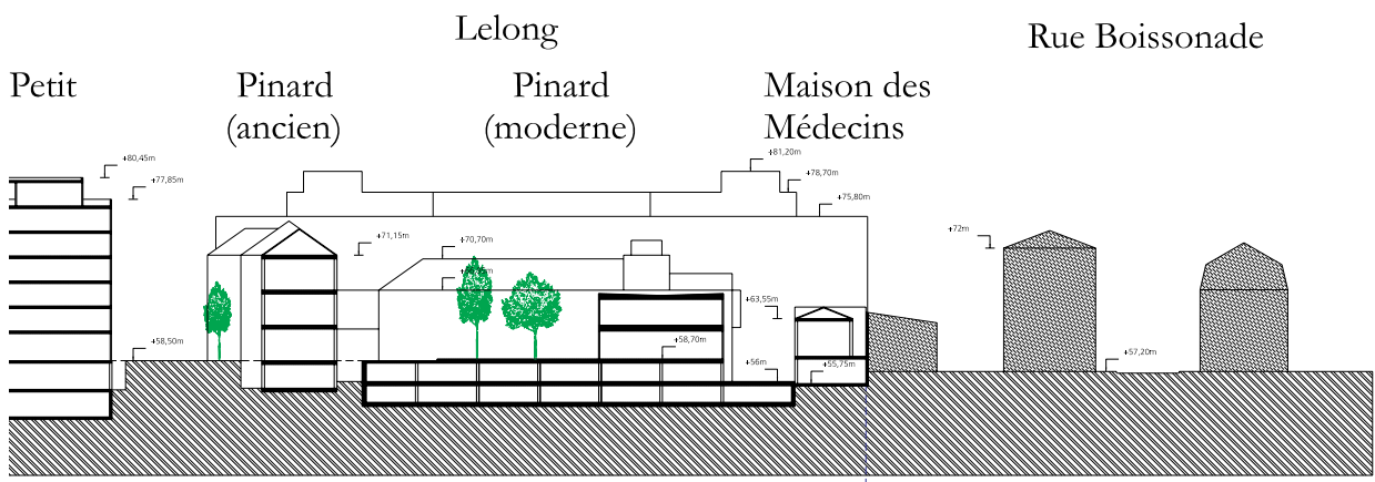
COUPE AA'
