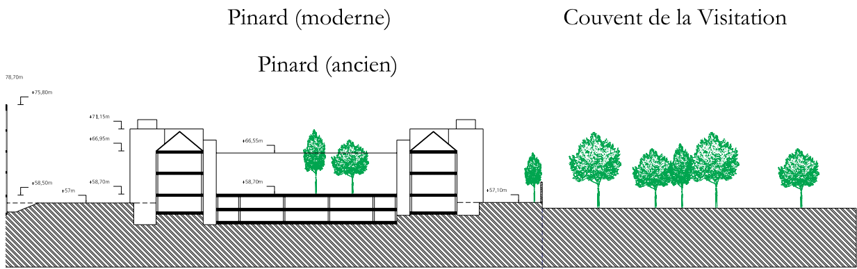
COUPE BB'
