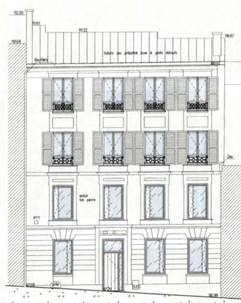
Élévation nord coté rue Levert - Etat projeté
