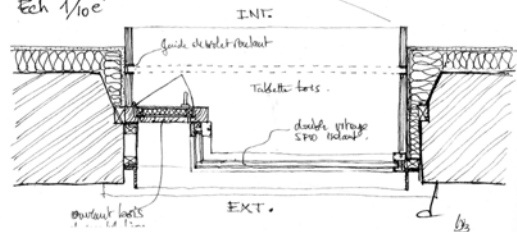
Détail en plan Ech 1/10e
