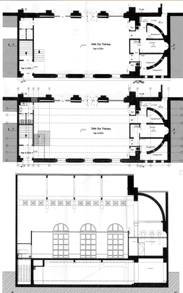
Ci-dessus, de haut en bas : vue intérieure de la chapelle ; plans et coupe du projet de la chapelle latérale, avec la conservation de l'abside (document G2A conception).
