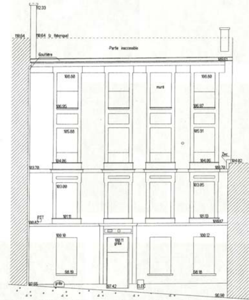
Élévation nord coté rue Levert - Etat actuel
