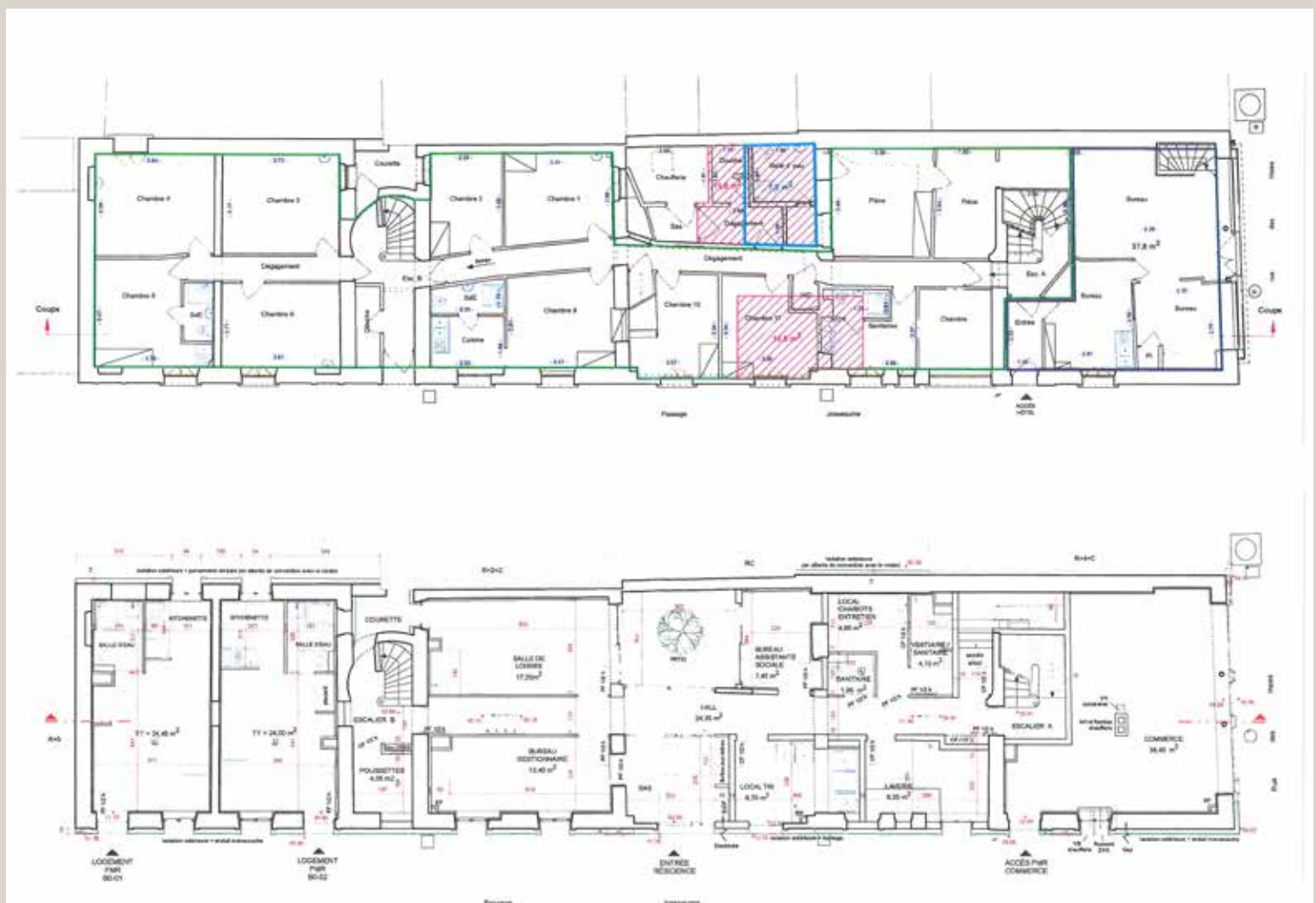
Plan du rez-de-chaussée, états existant (en haut) et projeté (en bas) (© Cabinet d'architecture Françoise Ruel).
