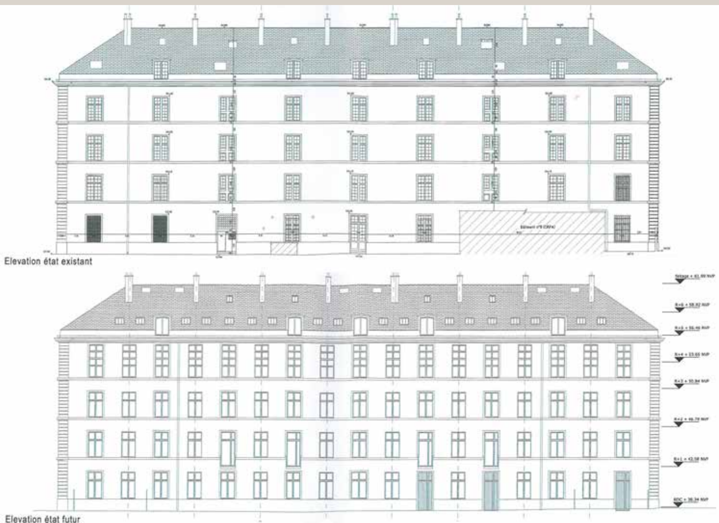
Élévation de la façade arrière du bâtiment A (aile gauche), états existant (en haut) et projeté (en bas) (© LIN Architectes Urbanistes / MIR Architectes).
