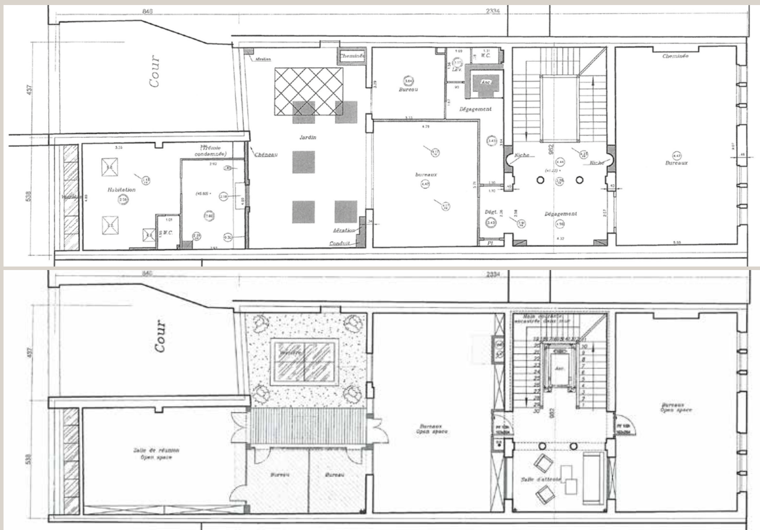
Plan du premier étage, repérage des démolitions (en haut) et état projeté (en bas) (© Bismut & Bismut).
