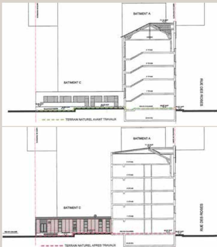
Coupe transversale, état existant (en haut) et premier projet (en bas) (© S.A. d'architecture Pierre et Cédric Vigneron & Partenaires).
