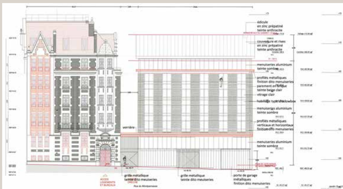
Élévation de la façade rue du Montparnasse, état projeté (© A-C. Perrot & F. Richard architectes).
