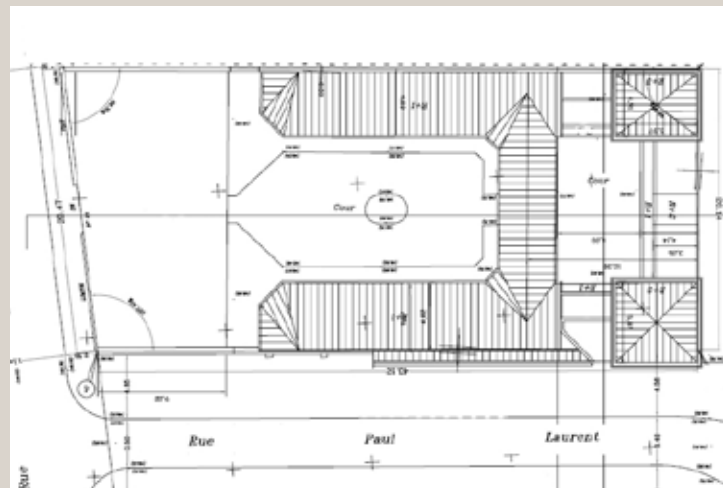
Plan de masse et de toiture, nouveau projet (© Ph. Belin architecte).
