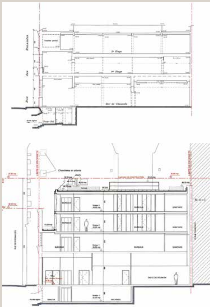
Coupe longitudinale, états existant (en haut) et projeté (en bas) (© DGM & Associés).
