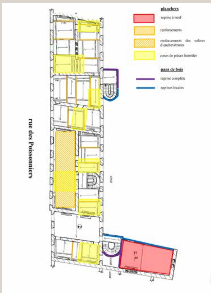
Plan d'un étage courant existant. Analyse structurelle des planchers et maçonneries existants (extrait du diagnostic structurel réalisé suite au vœu du 19 novembre 2015) (© Bureau Michel Bancon).
